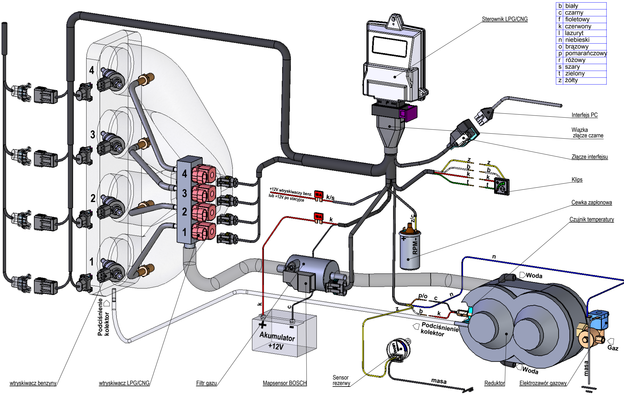
Rys. 1 Schemat podłączenia
