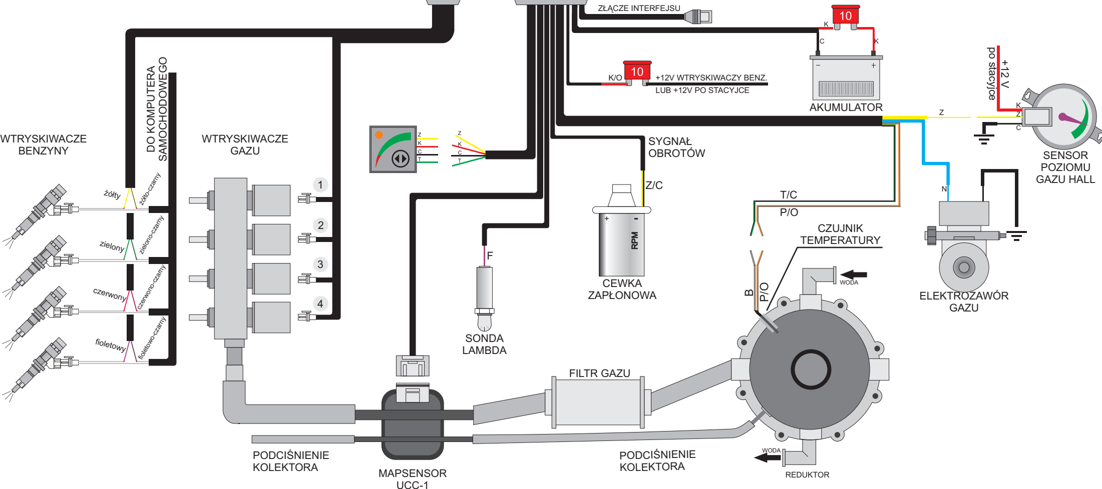
SCHEMAT PODŁĄCZENIA
